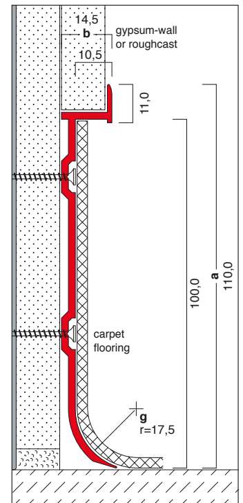
E6/U 110,0 x 14,5 mm
