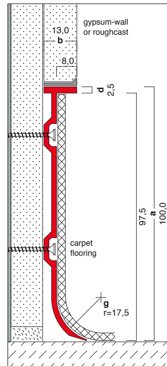
E4/U 100,0 x 13,0 mm
