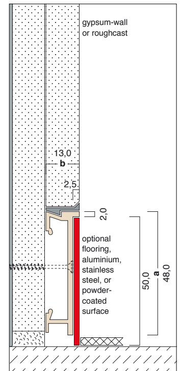
C21-A 48,0 x 13,0 mm
