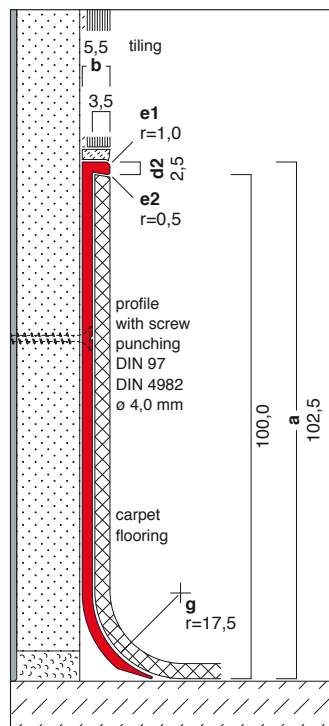
E1 102,5 x 5,5 mm
