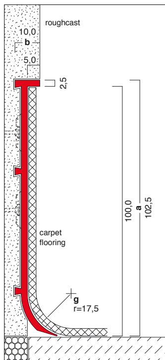
E5 102,5 x 10,0 mm
